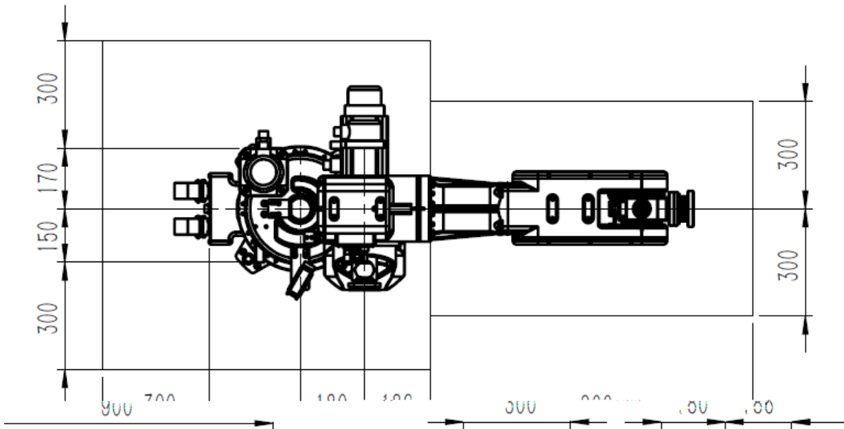
4.1 HSR-JR630-1800
